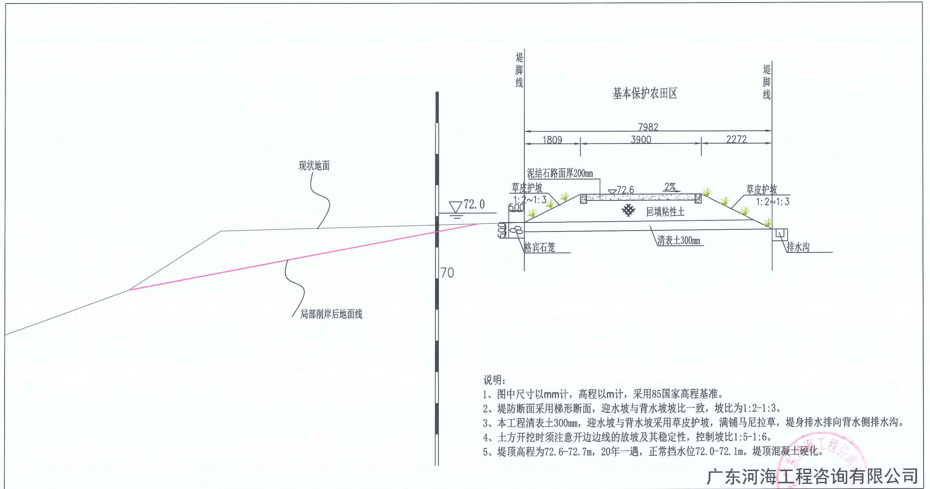
附件2.2 乳城镇前进村委会滩头村右岸河段整治工程典型断面图
